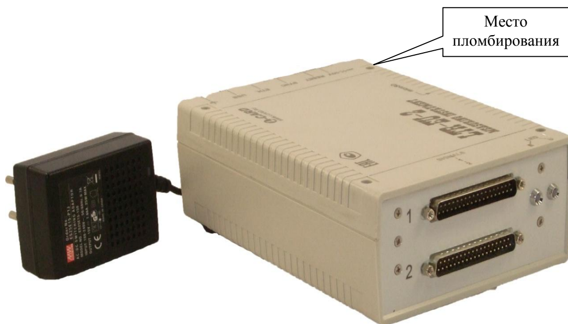
Рисунок 2 – Внешний вид установки измерительной LTR-EU-2-5
