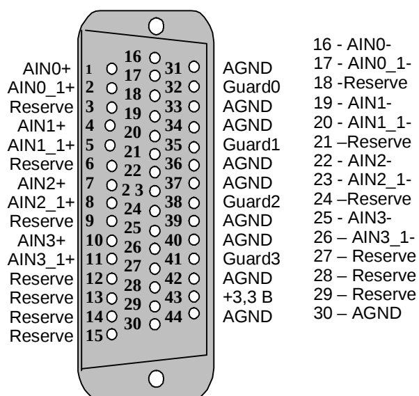
Разъем XP2 (вид спереди)
