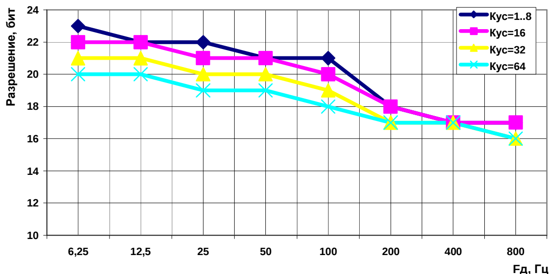
Зависимость разрешения от частоты дискретизации
