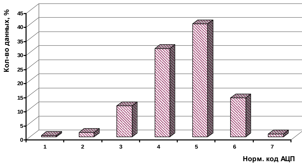
Гистограмма распределения при K_u=4 , F_d=6,25 Гц
