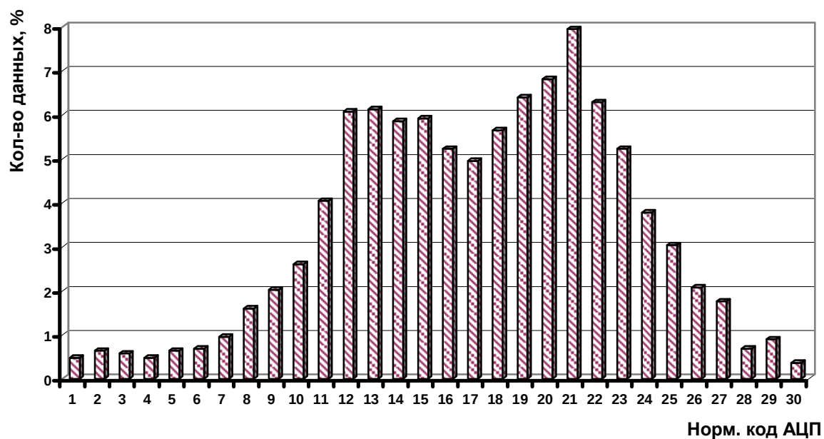
Гистограмма распределения при K_u=32 , F_d=6,25 Гц
