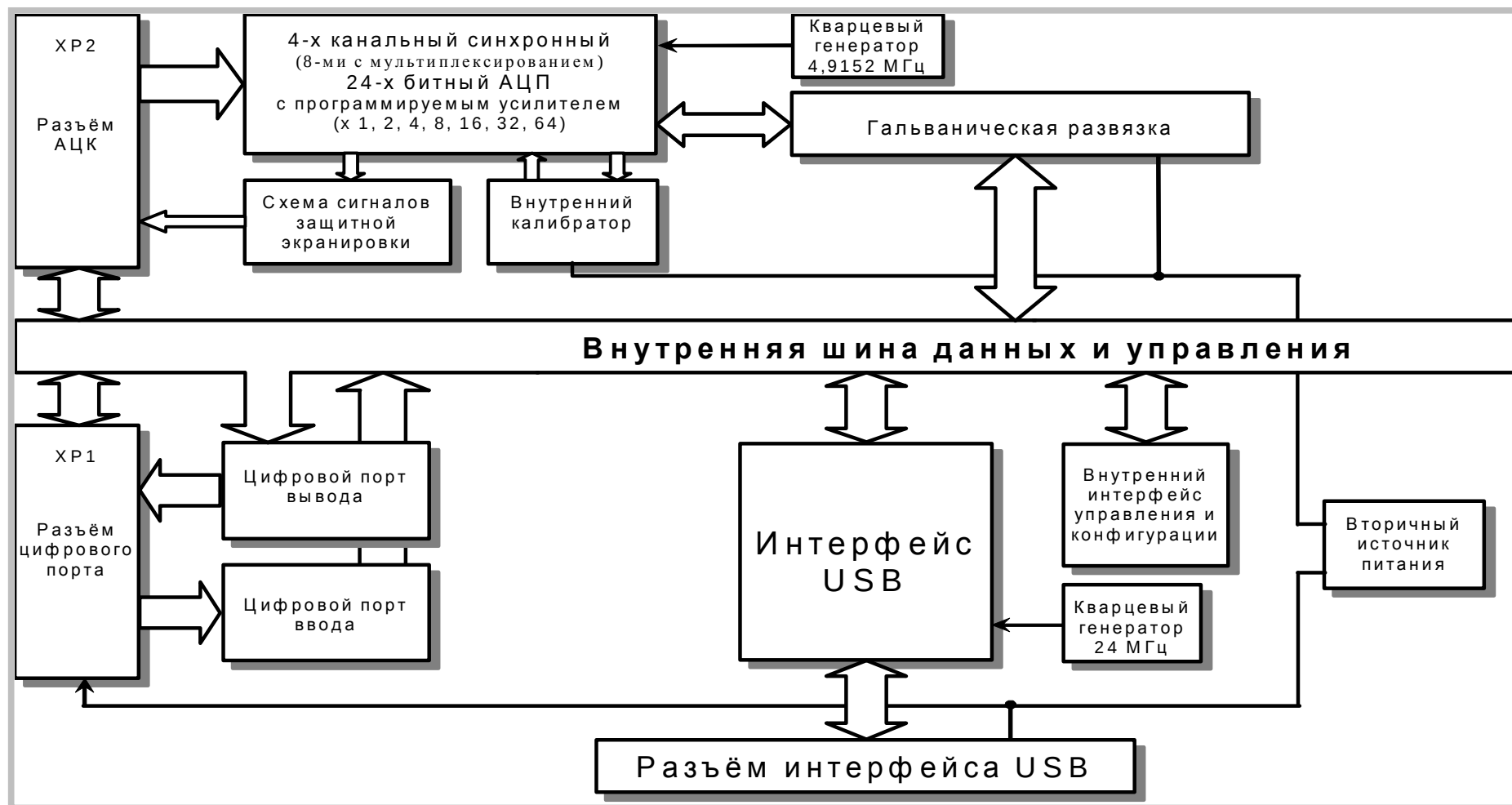
Функциональная схема ЛА-И24USB
